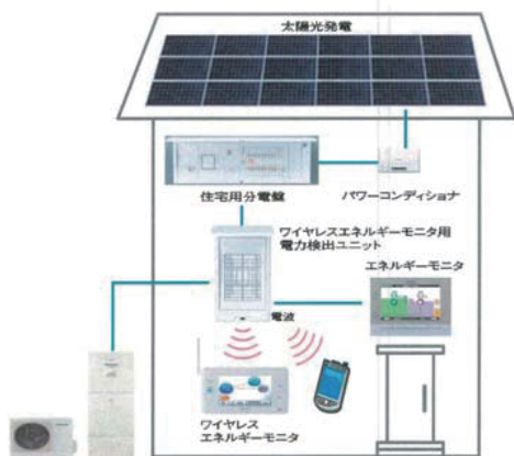
▲〈HEMSの略図〉太陽光発電と、各種家電をつなぎ使用電力と発電の電気をモニター確認することで、子供たちへの環境教育にもつながります。
